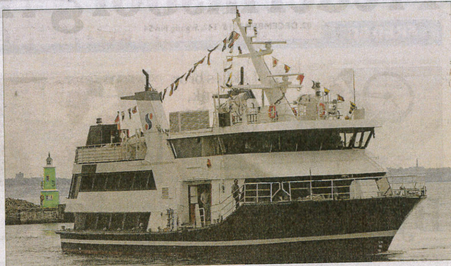
Firmaet Amminex A/S vil levere en kombineret løsning med partikelfiltre og NOx katalysatorer til skibet M/F Pernille, der sejler mellem Helsingør og Helsingborg. Fotos: Thomas Olsen
